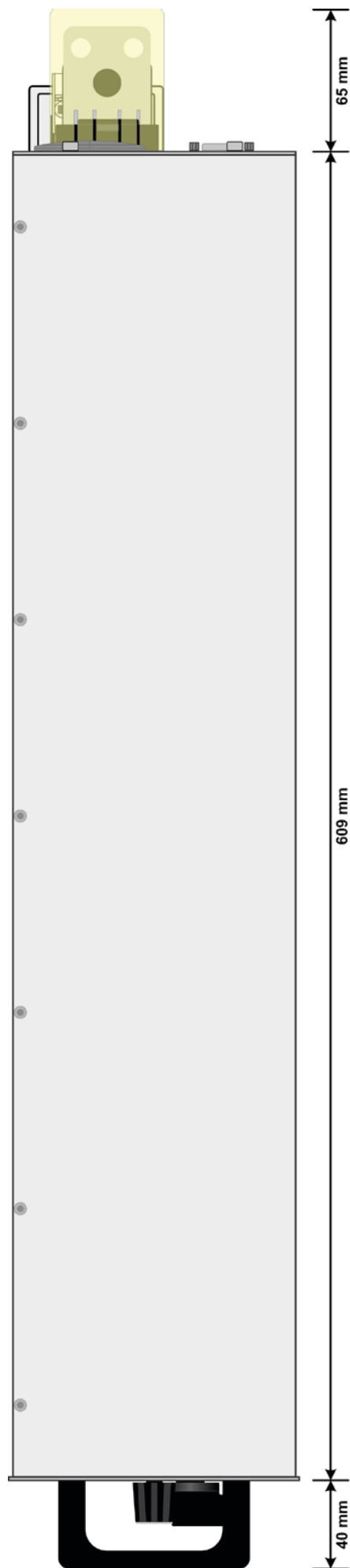
图 6 - 侧视图 (左边)
