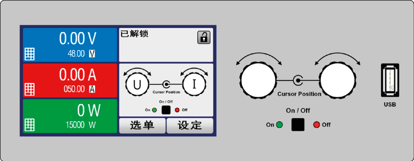
图 8 – 控制面板
