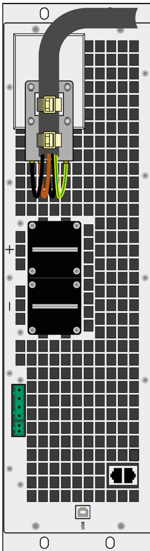
图 4 - 后视图 (PSI 9000从机)
