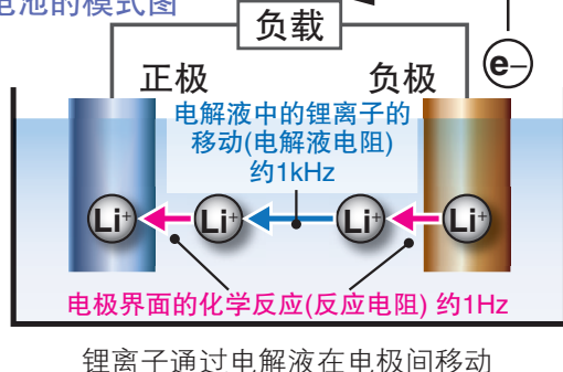
电池的模式图
