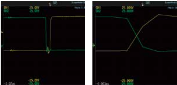
变频器门极信号波形(20kHz)
